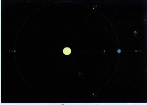
লাগ্রাঞ্জিয়ান পয়েন্ট
